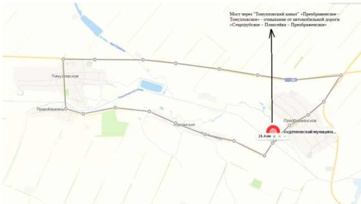
Рисунок 15- Схема объездной дороги в районе моста через Томузловский канал на автомобильной дороге «Преображенское - Томузловское» - отмыкание от автомобильной дороги «Стародубское – Плаксейка – Преображенское» с.Преображенское
